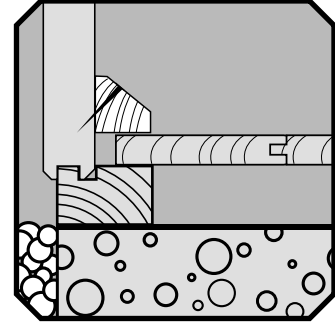
Plinten aan de wand spijkeren. Fußleisten an der Wand festnageln. Nail the skirting boards to the wall.
