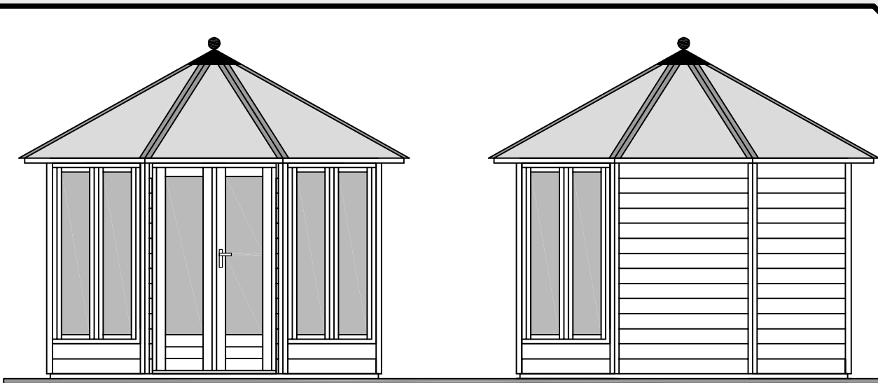
Voor aanzicht Vorder ansicht Front view
