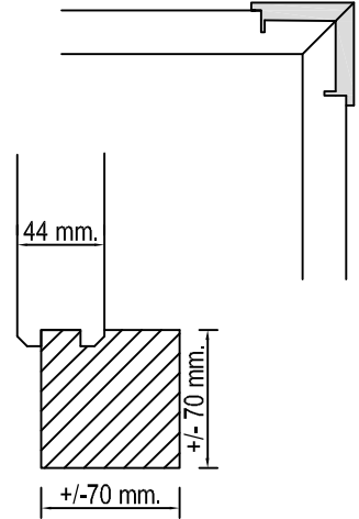
A - A
