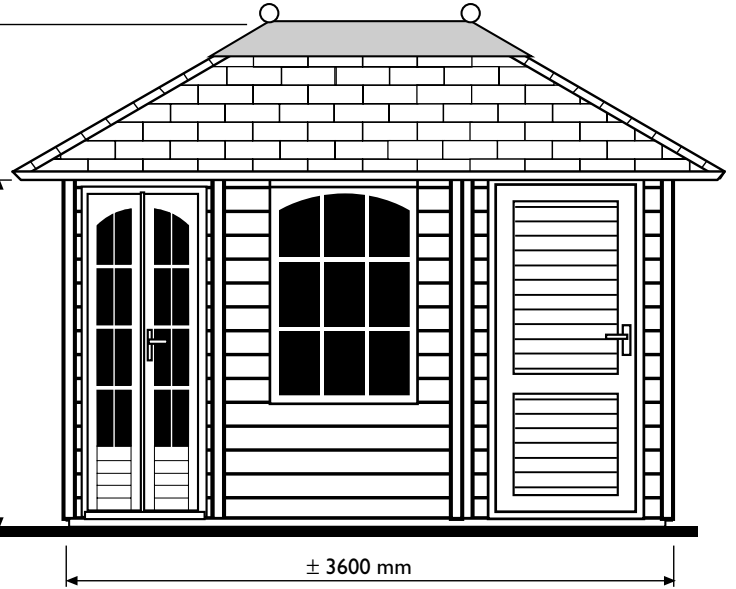
Zij aanzicht Seiten Ansicht Side view
