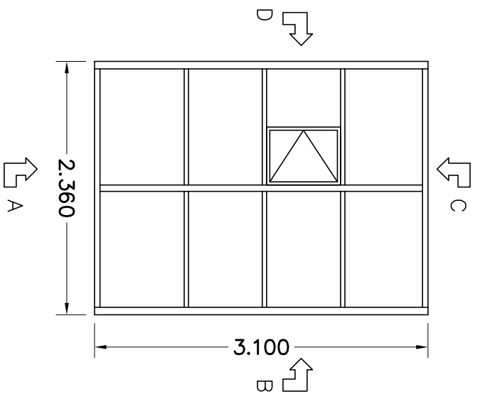
BOVENAANZICHT
