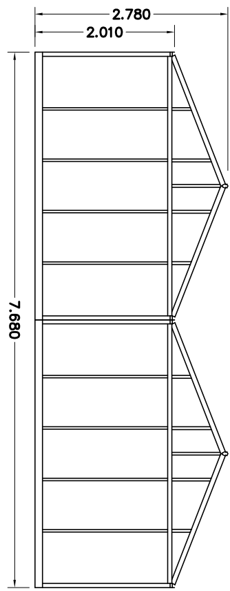
AANZICHT A
