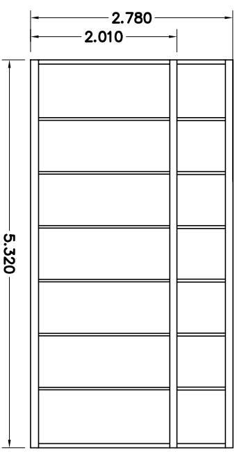
AANZICHT B
