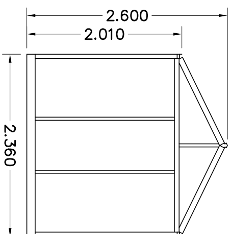
AANZICHT A
