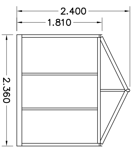
AANZICHT C
