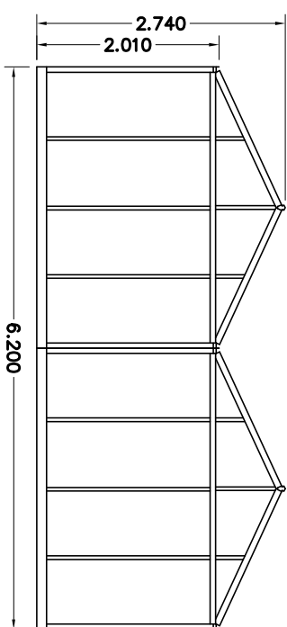
AANZICHT A
