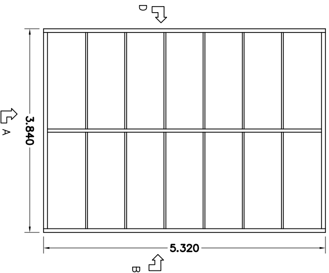
BOVENAANZICHT
