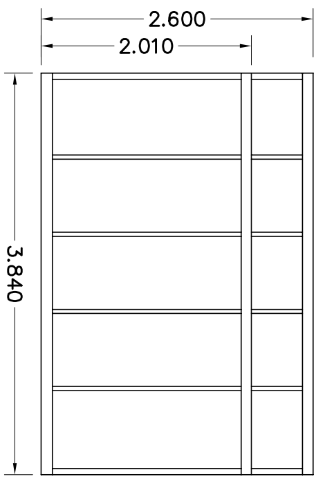
AANZICHT B
