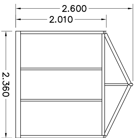
AANZICHT C
