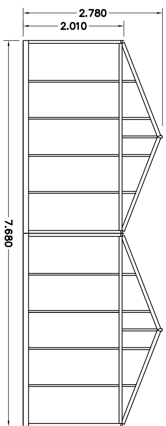
AANZICHT C
