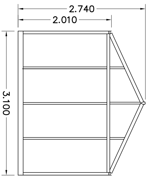
AANZICHT C
