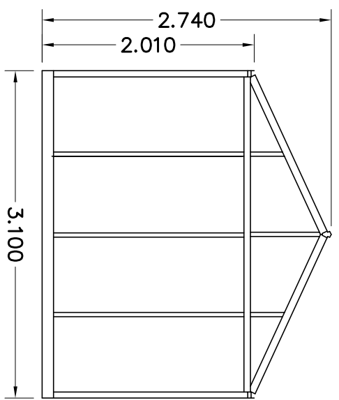
AANZICHT A
