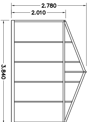
AANZICHT A
