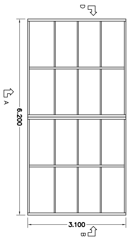
BOVENAANZICHT
