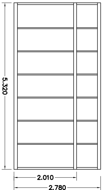
AANZICHT D
