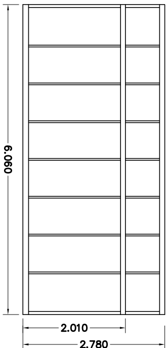
AANZICHT D
