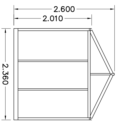
AANZICHT C
