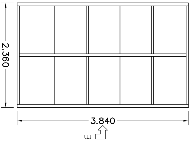
BOVENAANZICHT
