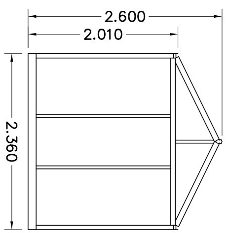
AANZICHT A
