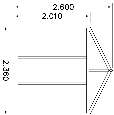
AANZICHT A
