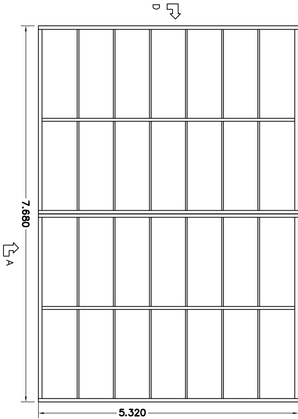
BOVENAANZICHT
