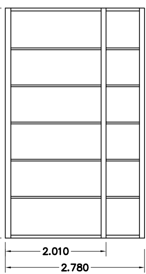
AANZICHT D
