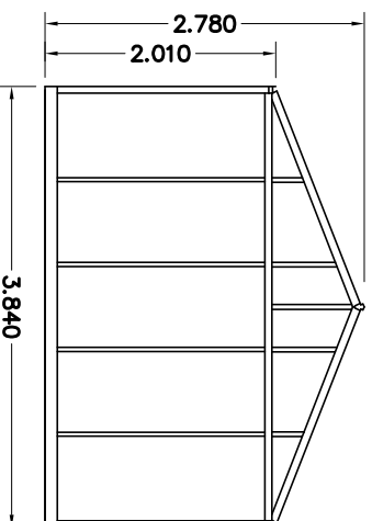
AANZICHT C
