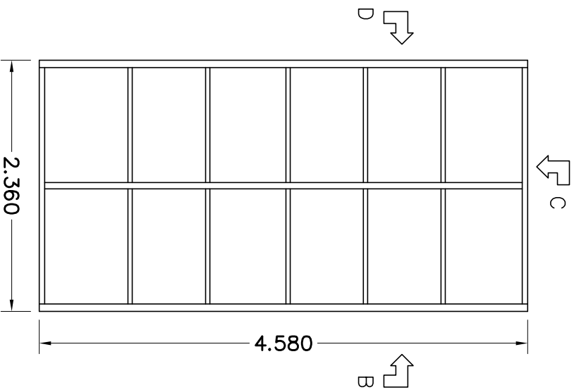
BOVENAANZICHT
