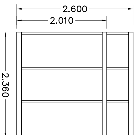
AANZICHT B
