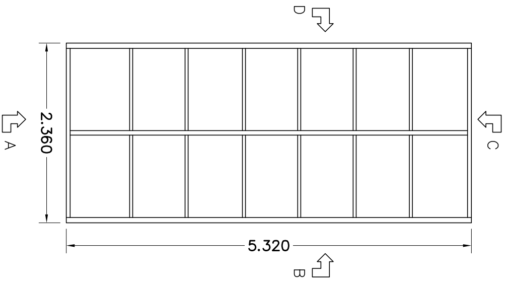
BOVENAANZICHT
