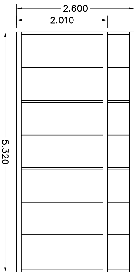
AANZICHT B
