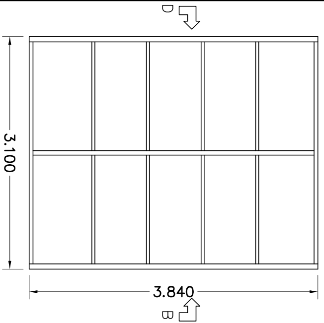
BOVENAANZICHT C
