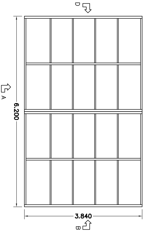
BOVENAANZICHT
