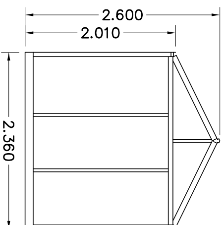
AANZICHT C
