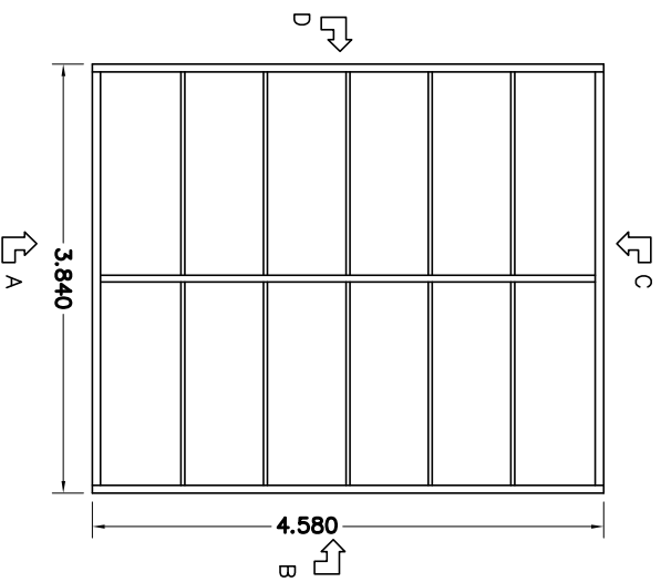
BOVENAANZICHT
