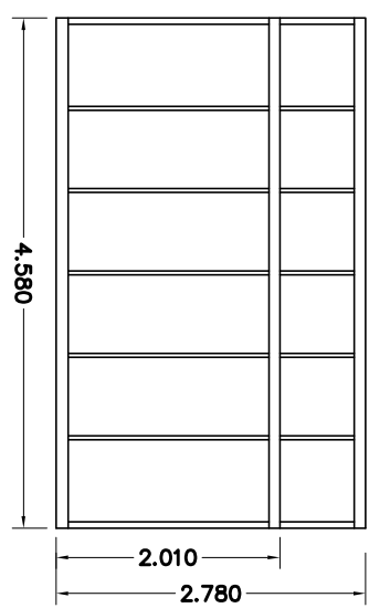
AANZICHT D
