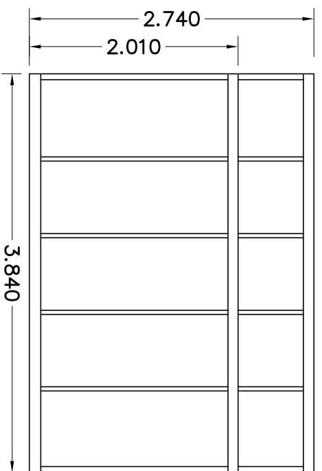
AANZICHT D
